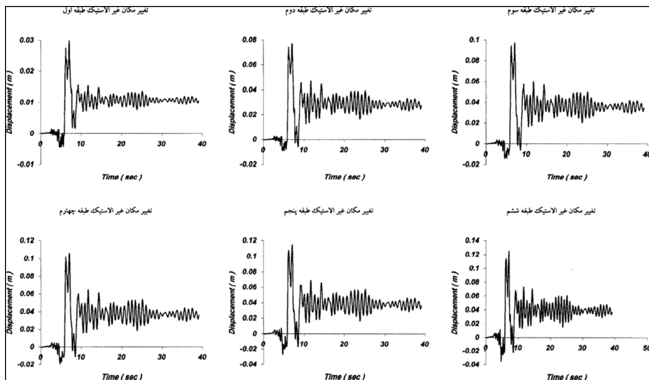
شکل ۸. جابجایی غیرالاستیک هر یک از طبقات قاب مفصلی ۶ طبقه در اثر زمین لرزه السنترو
