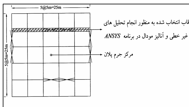
شکل ۴. هندسه پلان ساختمان‌های با سیستم قاب مفصلی با مهاربندهای هم محور
