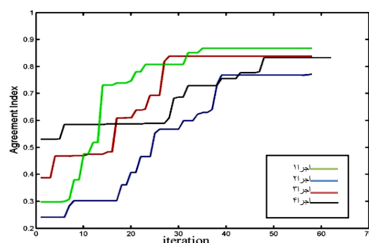
شکل ۵. منحنی‌های همگرایی الگوریتم اکستریمال مجموعه داده ۶×۶ اول
