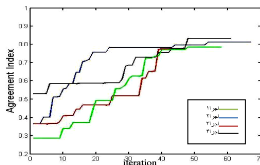
شکل ۶. منحنی‌های همگرایی الگوریتم اکستریمال مجموعه داده ۶×۶ دوم
