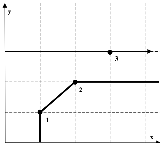
شکل ۵. مرز کارایی پس از حذف واحد ۳ برای مثال ۴.
