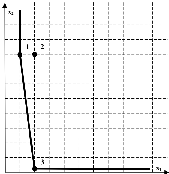
شکل ۱. واحدهای تحت مطالعه و مرز کارایی برای مثال ۱.
