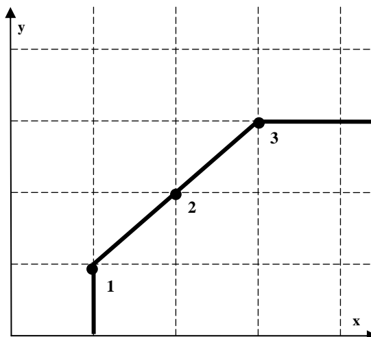
شکل ۴. واحدهای تحت مطالعه و مرز کارایی برای مثال ۴.
