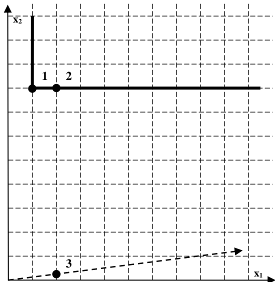
شکل ۲. مرز کارایی پس از حذف واحد ۳ برای مثال ۱.
